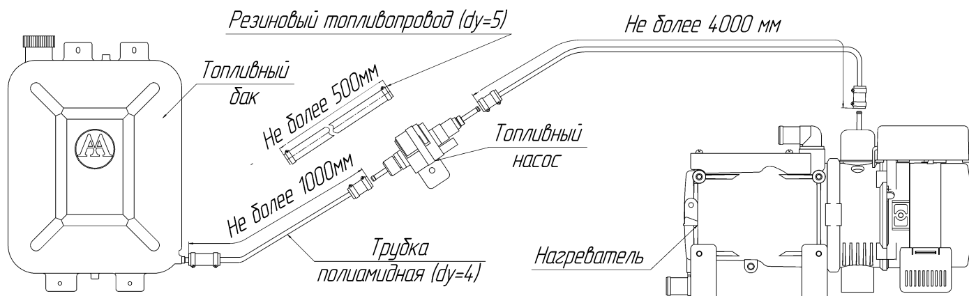
Рис. 9- Схема присоединения топливопровода к узлам подогревателя
